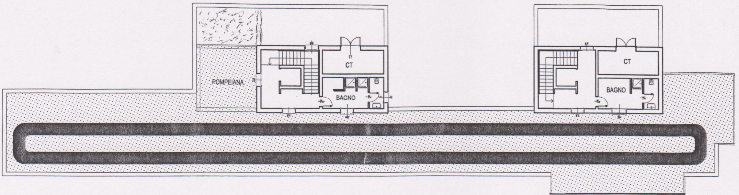
PALAZZO ILLINOIS BLOCCO B ED A PIANO QUINTO COMPOSTO DA GIARDINO PENSILE, SPOGLIATOI CON DOCCE E WC, POMPEIANA, PISTA JOGGING E CENTRALI TERMICHE scala 1:200
